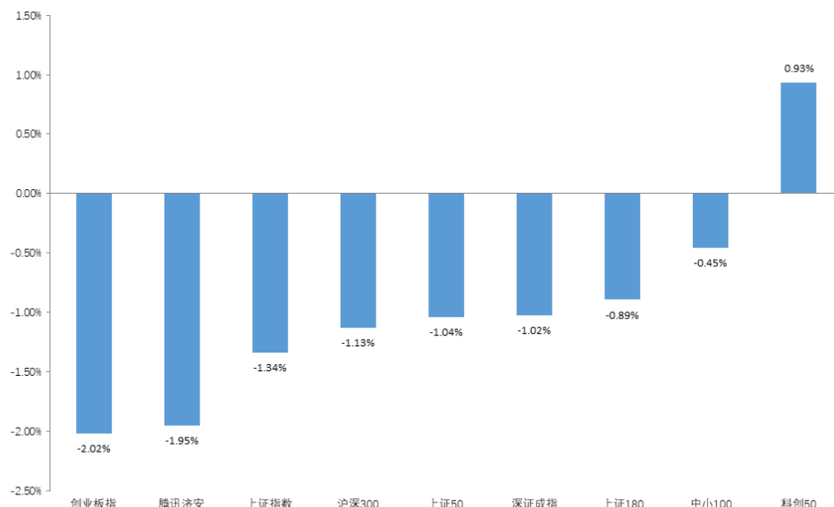
图 1：指数动态（2025.01.06—2025.01.10）
