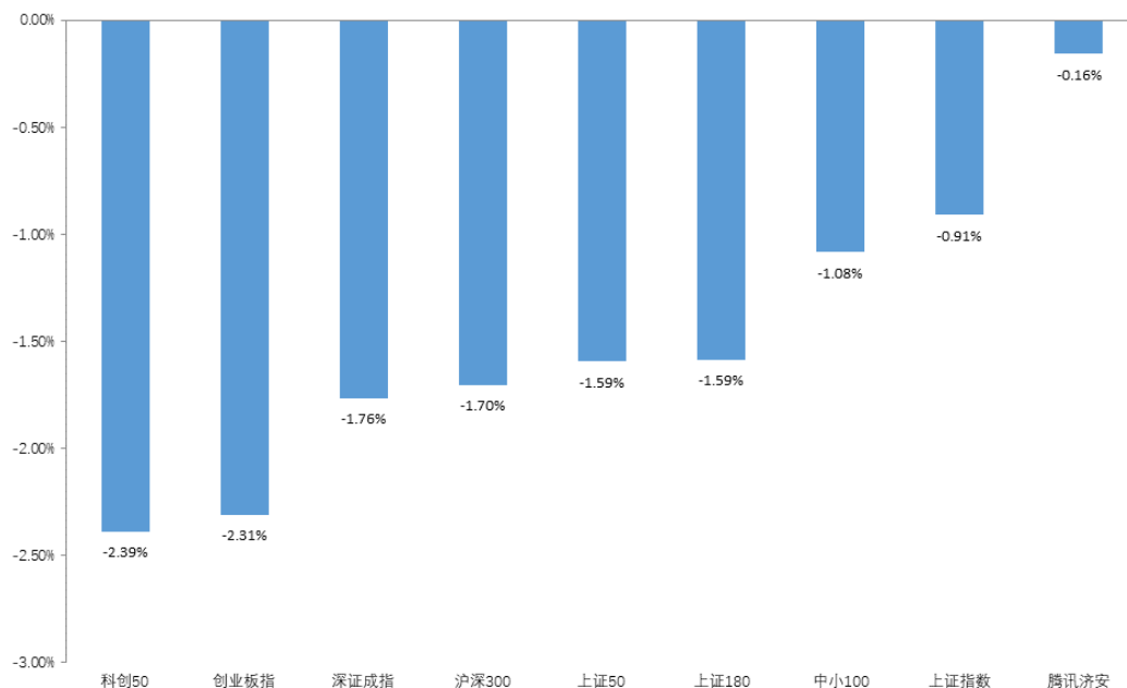
图 1：指数动态（2023. 12. 11—2023. 12. 15）
