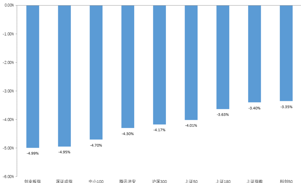
图 1：指数动态（2023. 10. 16—2023. 10. 20）
