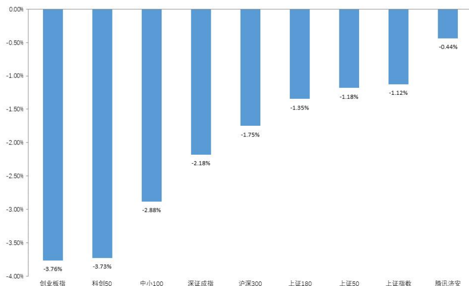
图 1：指数动态（2023.02.13—2023.02.17）
