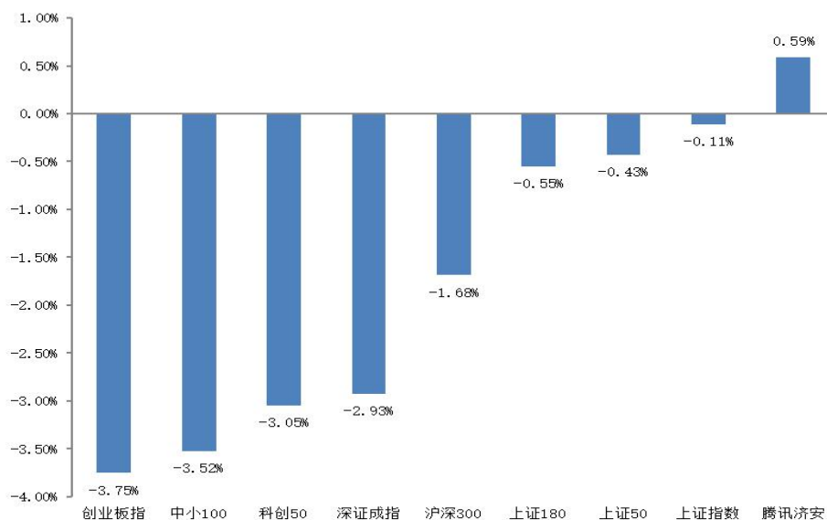
图 1：指数动态（2022.02.28—2022.03.04）
