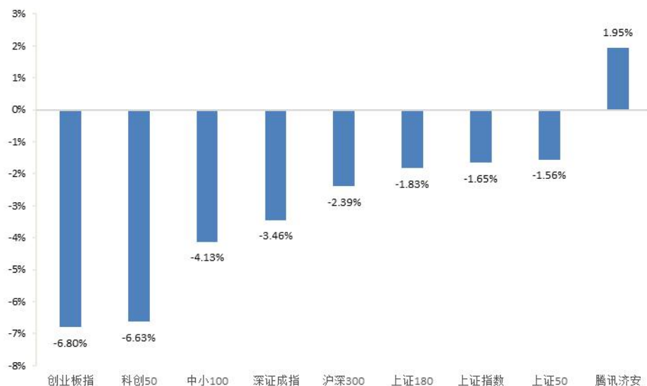
图 1：指数动态（2022.01.04—2022.01.07）
