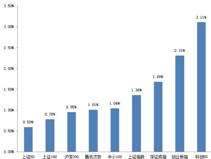
图 1：指数动态（2021.11.08—2021.11.12）
