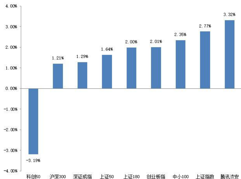
图 1：指数动态（2021.08.23—2021.08.27）
