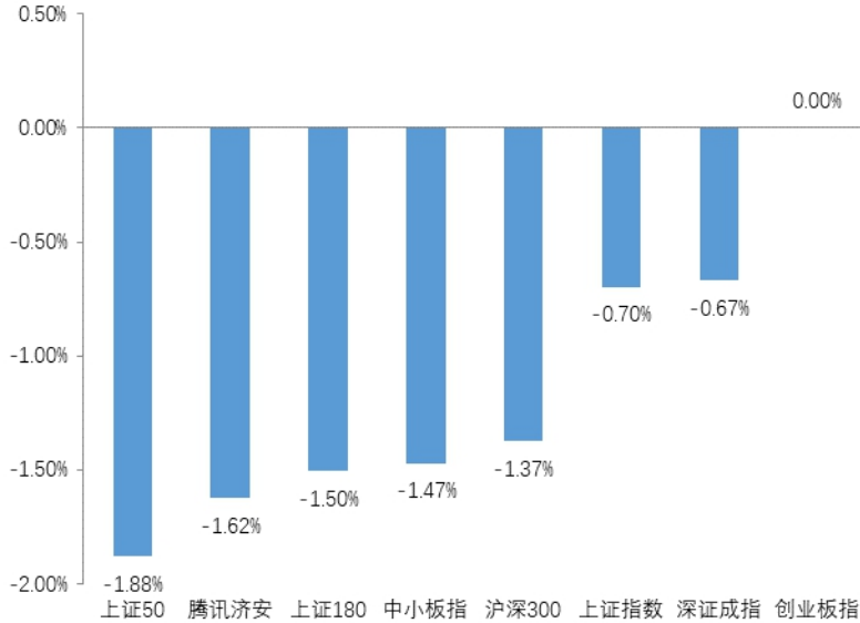
图 1：指数动态（2021.04.12—2021.04.16）
