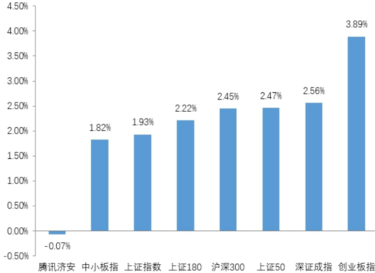
图 1：指数动态（2021.03.29—2021.04.02）
