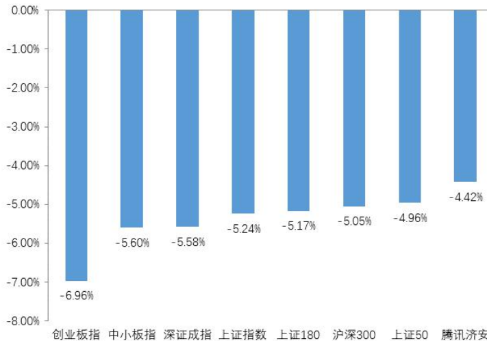
图 1：指数动态（2020.02.24—2020.02.28）
